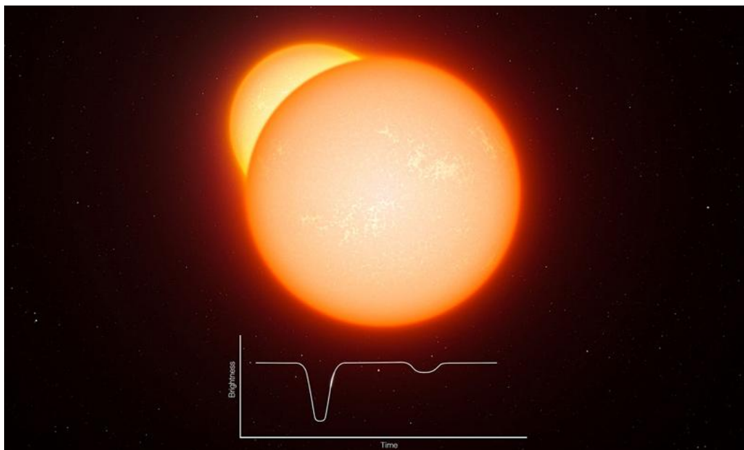
Umělecká představa zákrytové dvojhvězdy se světelnou křivkou. Zdroj: ESO
