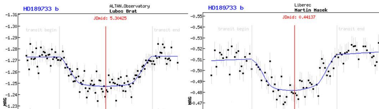
Dvě světelné křivky tranzitu exoplanety HD189733 b. Vlevo pořízená pomocí CCD kamery SBIG ST-8 (L. Brát) vpravo pomocí digitální zrcadlovky Canon EOS 1000D (M. Mašek).
